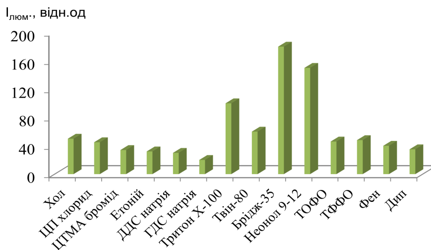
Рис. 5. Вплив ПАР та ДАД на інтенсивність люмінесценції сорбату комплексу Sc(III)-ресвератролу; ( C_{\text{Sc(III)}} = 5 \cdot 10^{-3} моль/л, C_{\text{ресв}} = 1 \cdot 10^{-5} моль/л).
