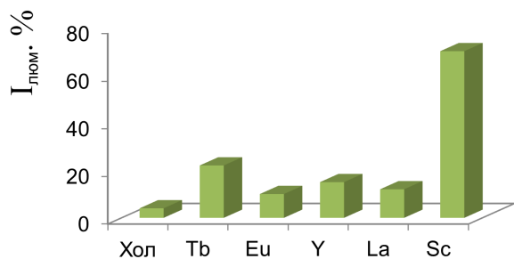
Рис. 3. Відносна інтенсивність люмінесценції ресвератролу у твердій фазі в присутності різних йонів металів; ( C_{\text{Ln}} = 1 \cdot 10^{-3} моль/л; C_{\text{ресв}} = 1 \cdot 10^{-5} моль/л).
