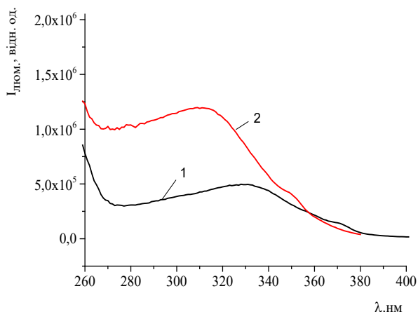
Рис. 2. Спектр збудження люмінесценції розчину ресвератролу (1) та комплексу \text{Sc(III)} – ресвератрол; ( C_{\text{ресв}} = 1 \cdot 10^{-5} моль/л, C_{\text{Sc(III)}} = 5 \cdot 10^{-3} моль/л).
