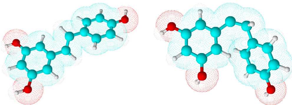
Рис.1. Структурні форми ресвератролу: 3,5,4'-тригідрокси-транс-ресвератрол (А) та 3,5,4'-тригідрокси-цис-ресвератрол (В).
