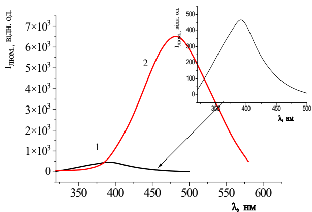
Рис. 4. Спектри люмінесценції розчину ресвератролу (1) та сорбату комплексу Sc(III)-ресвератролу на Silicagel Merk L100/160; ( C_{\text{Sc(III)}} = 5 \cdot 10^{-3} моль/л, C_{\text{ресв}} = 1 \cdot 10^{-5} моль/л).
