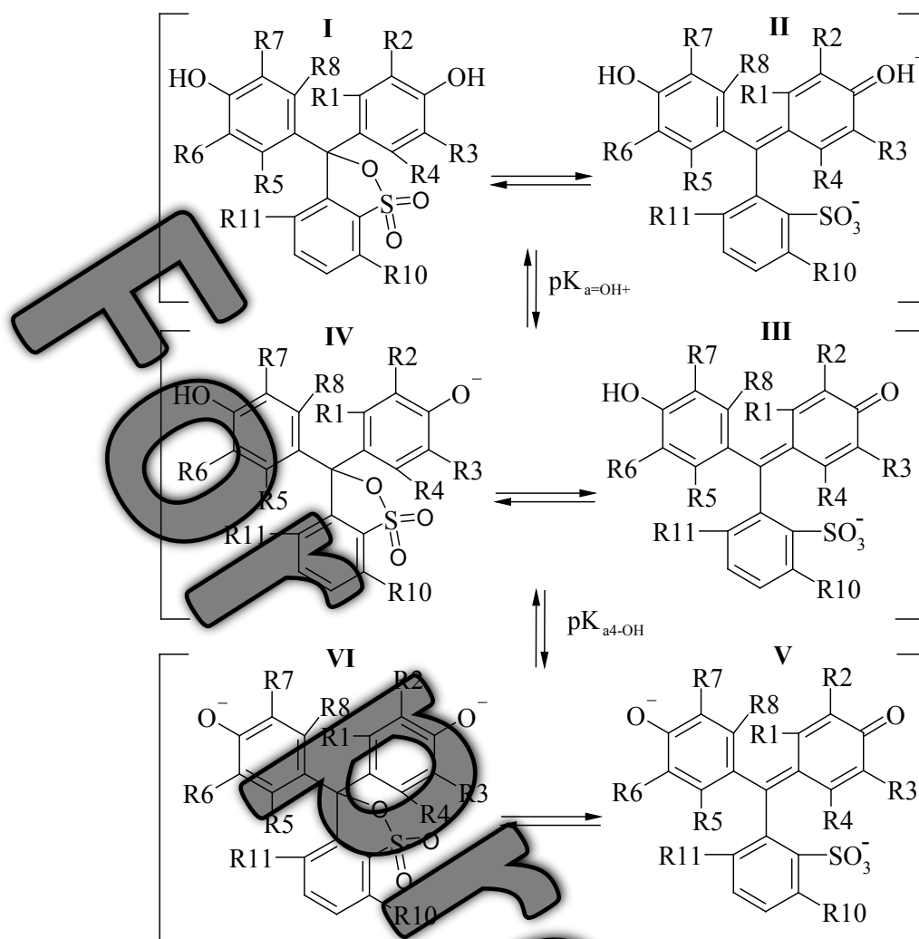
Схема 1. Кислотно-основные и таутомерные равновесия в растворах трифенилметановых красителей.
