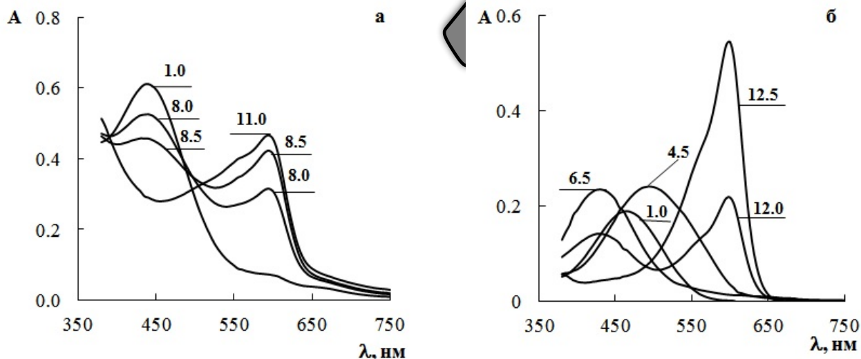
Рис. 5. Электронные спектры поглощения: а) пирокатехиновый фиолетовый (8); б) хромазурол S (10); C_{ТФК} = 2 \cdot 10^{-5} моль/дм 3 ; l = 1 см; числа на кривых соответствуют значениям pH среды.
